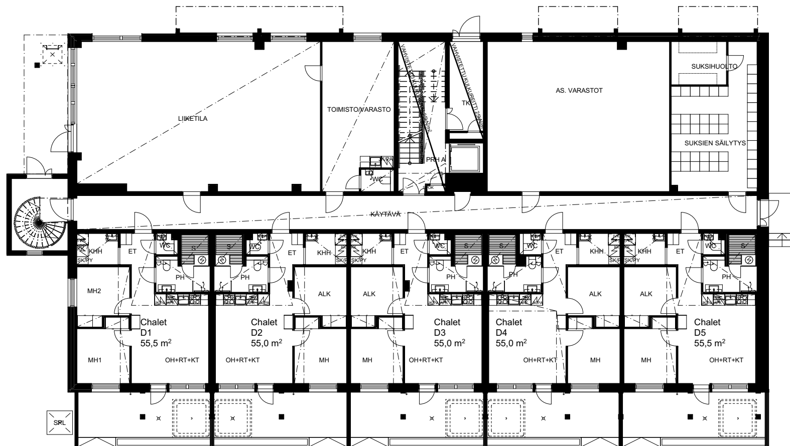
Kerros pohja 1. krs, 1:200
